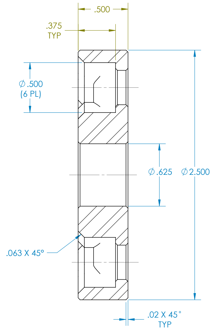
SECTION A-A SCALE 2 : 1
